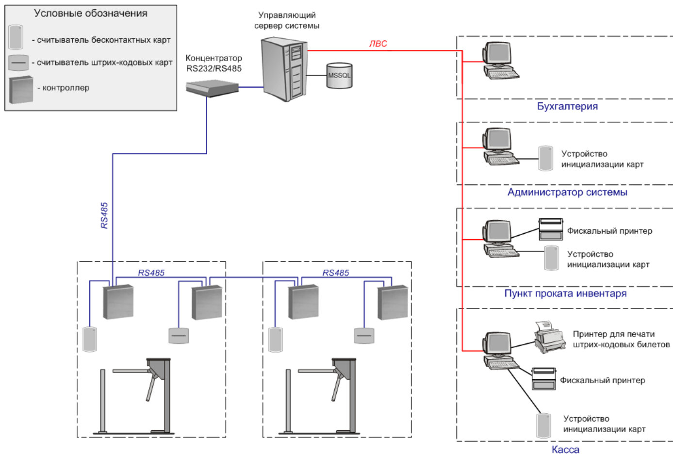
Структурная схема системы платного доступа "STOP-Cash"
