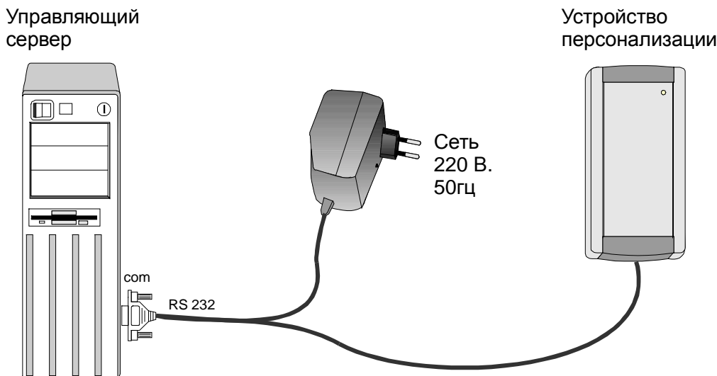
рис.1. Подключение устройства персонализации
